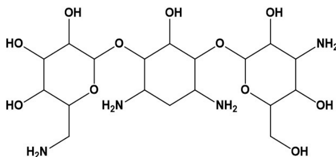
Kanamycin (KANA)
