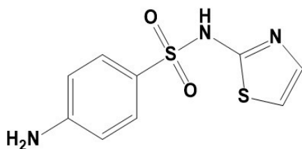
Sulphathiazole (SFZ)
